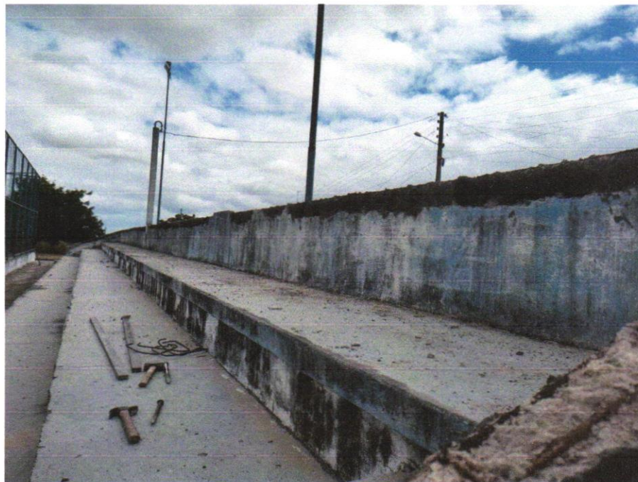
Foto 01 - Demolição de alvenaria de bloco de concreto de vedação
